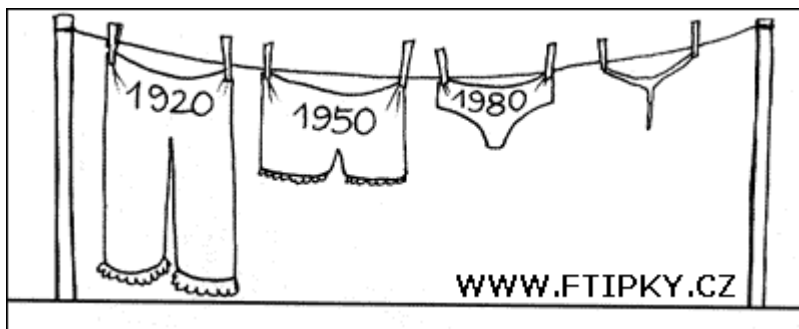
Důkaz stabilního oteplování zeměkoule
